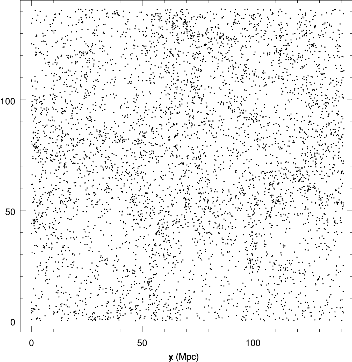
Spiral Galaxies (sfr > 1) - 5186 galaxies
