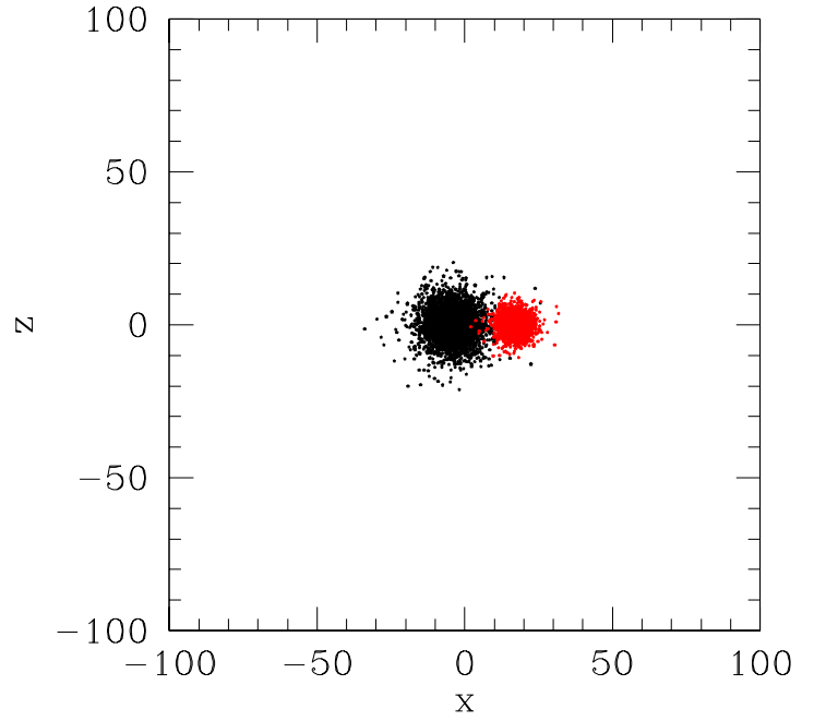
Galaxy pair 7m : step 1
