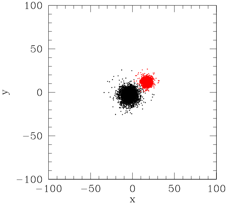
Galaxy pair 7m : step 1
