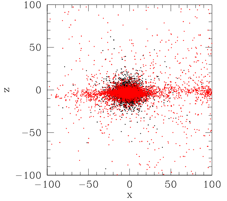
Galaxy pair 2m : step 50
