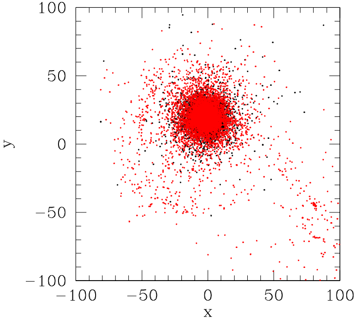
Galaxy pair 2m : step 50
