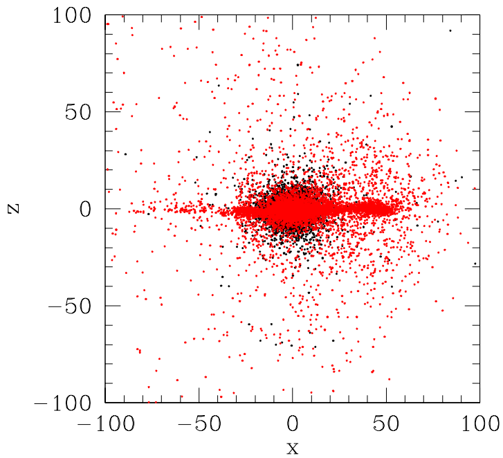
Galaxy pair 1m : step 15
