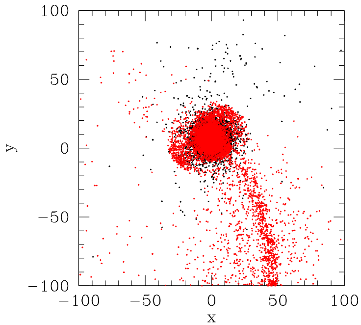
Galaxy pair 1m : step 15
